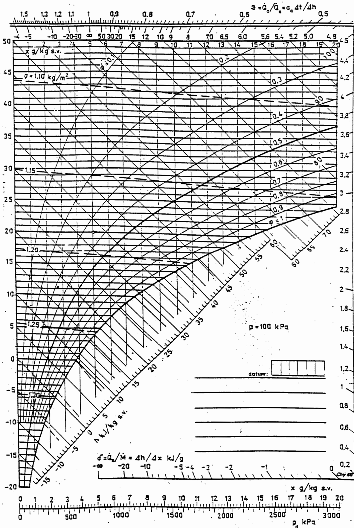
Đbr. 2.1 Mollierův h-x diagram
