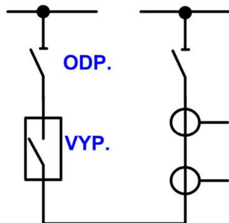
PODÉLNÝ SPÍNAČ
