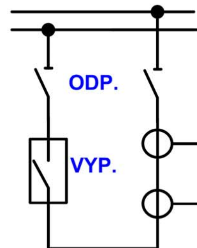
PŘÍČNÝ SPÍNAČ
