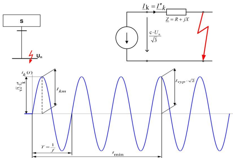
Obr.5 Elektricky vzdálený zkrat bez vzniku stejnosměrné složky
