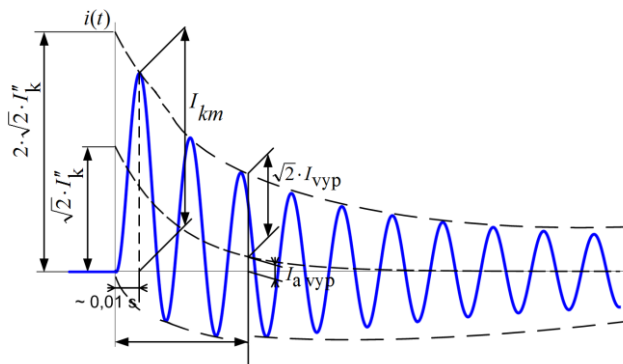
Obr.7 Zkrat elektricky blízký synchronnímu stroji
