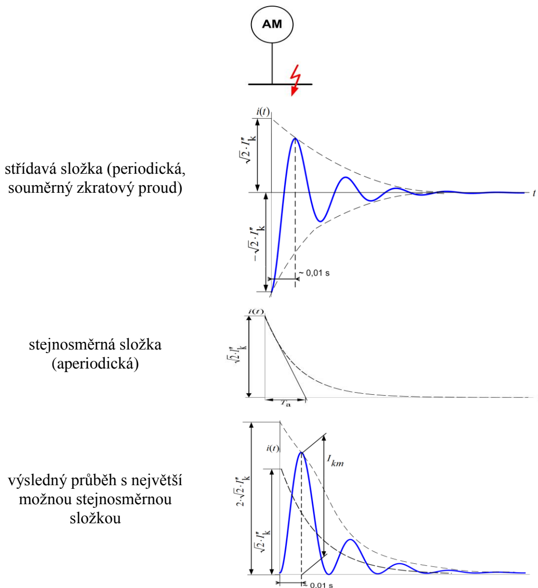
Obr.8 Zkrat na svorkách asynchronního motoru
