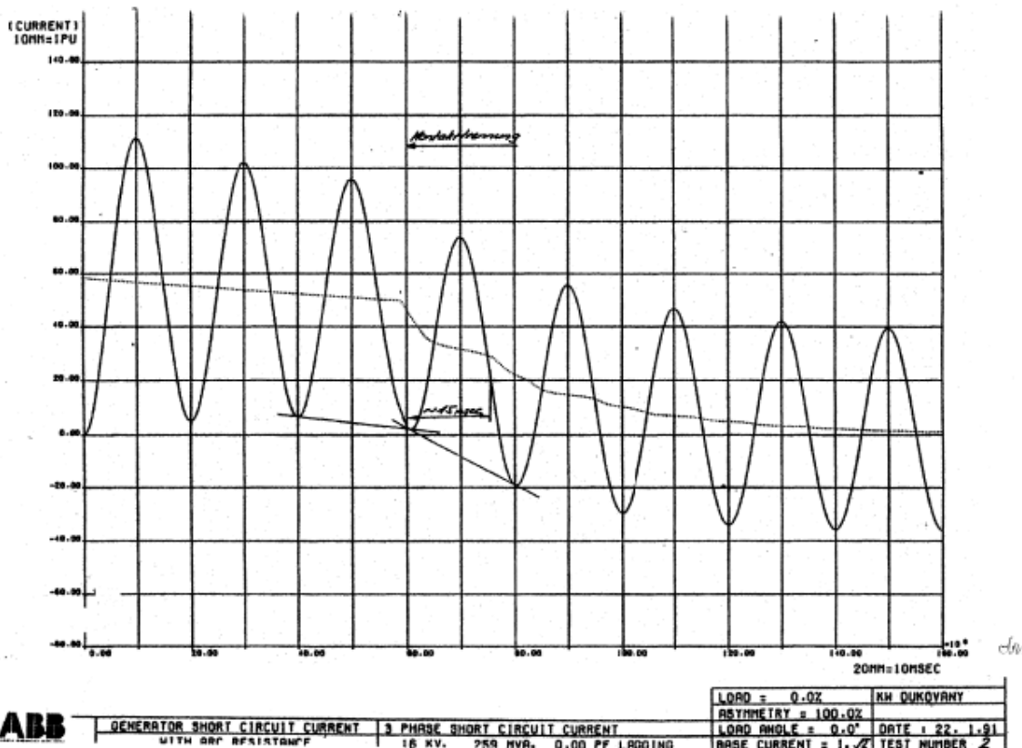
Obr.3 Příklad výsledku výpočtu průběhu zkratového proudu ve vývodu generátoru
