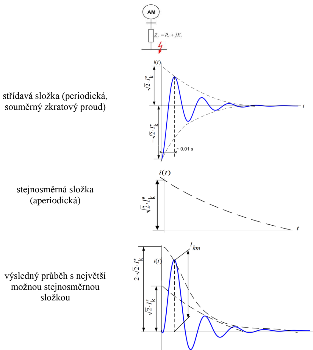
Obr.9 Zkratový příspěvek asynchronního motoru při zkratu za vnější impedancí Z_V
